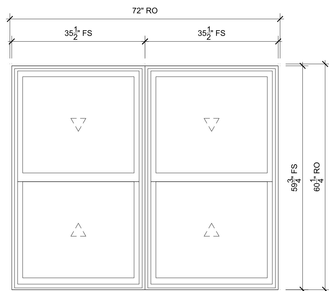
REAR - BEDROOM SCALE: 3/4" = 1'-0"
