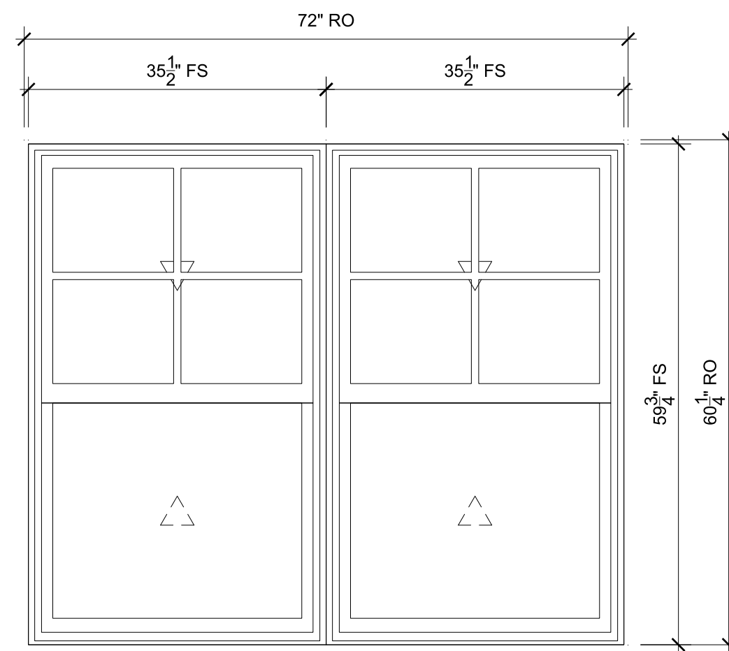
FRONT - BEDROOM SCALE: 3/4" = 1'-0"
