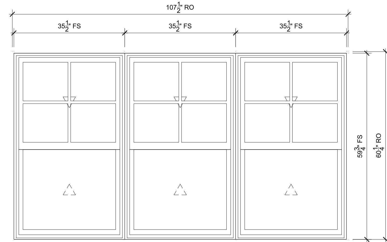
RIGHT - BONUS ROOM SCALE: 3/4" = 1'-0"
