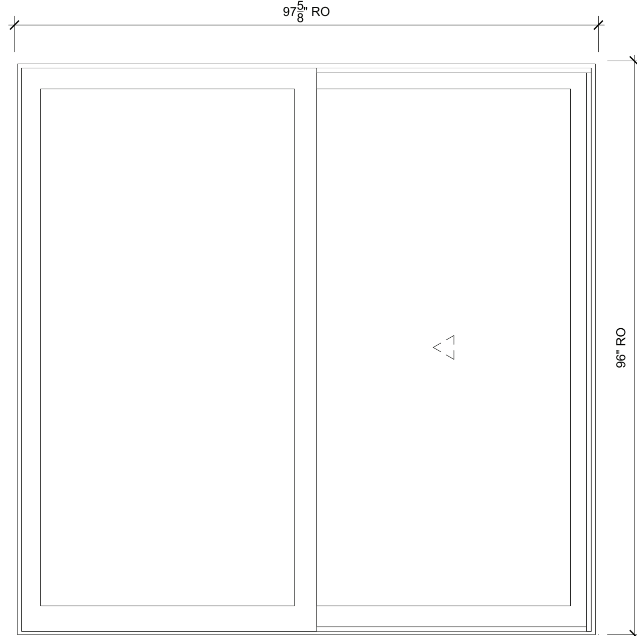
NORTH A1 & A2 SCALE: 3/4" = 1'-0"
