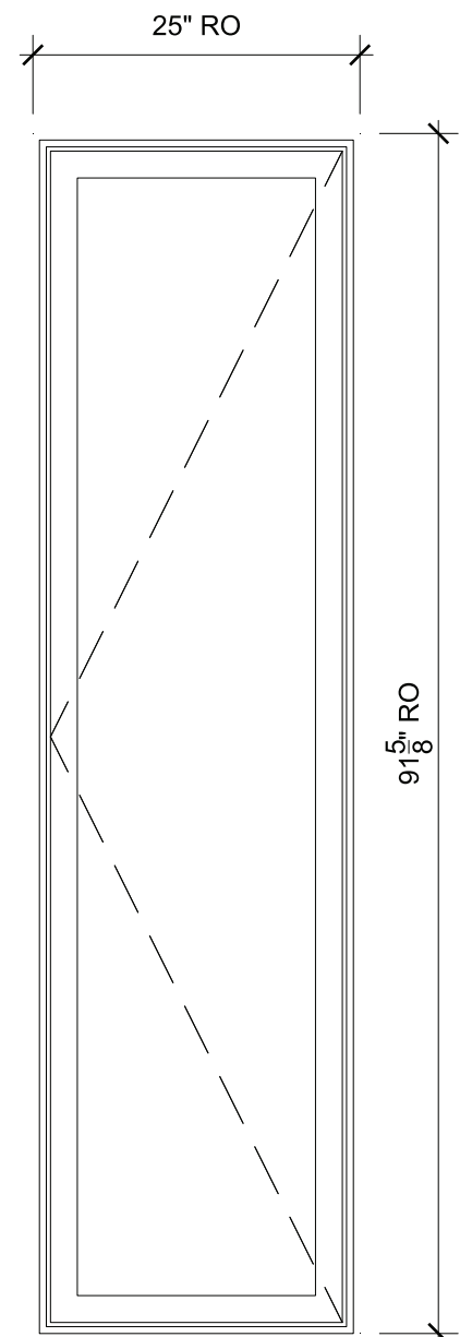
EAST O SCALE: 3/4" = 1'-0"
