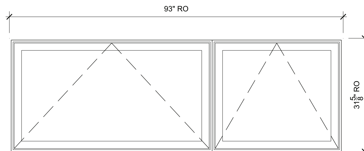
SOUTH R/Y SCALE: 3/4" = 1'-0"
